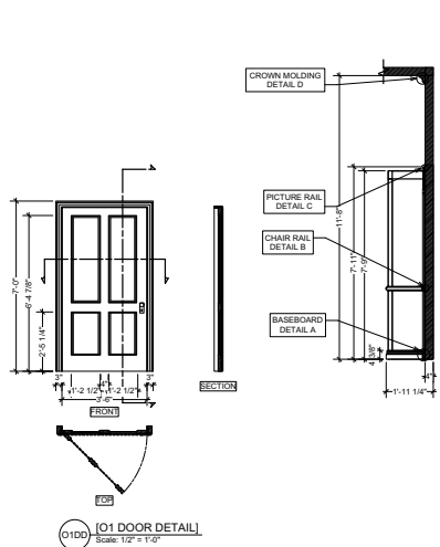
O1DO [O1 DOOR DETAIL] Scale: 1/2" = 1'-0"
