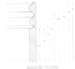
10 [DETAIL A] Scale: Actual Size
