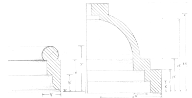
O8 [DETAIL C] Scale: Actual Size
