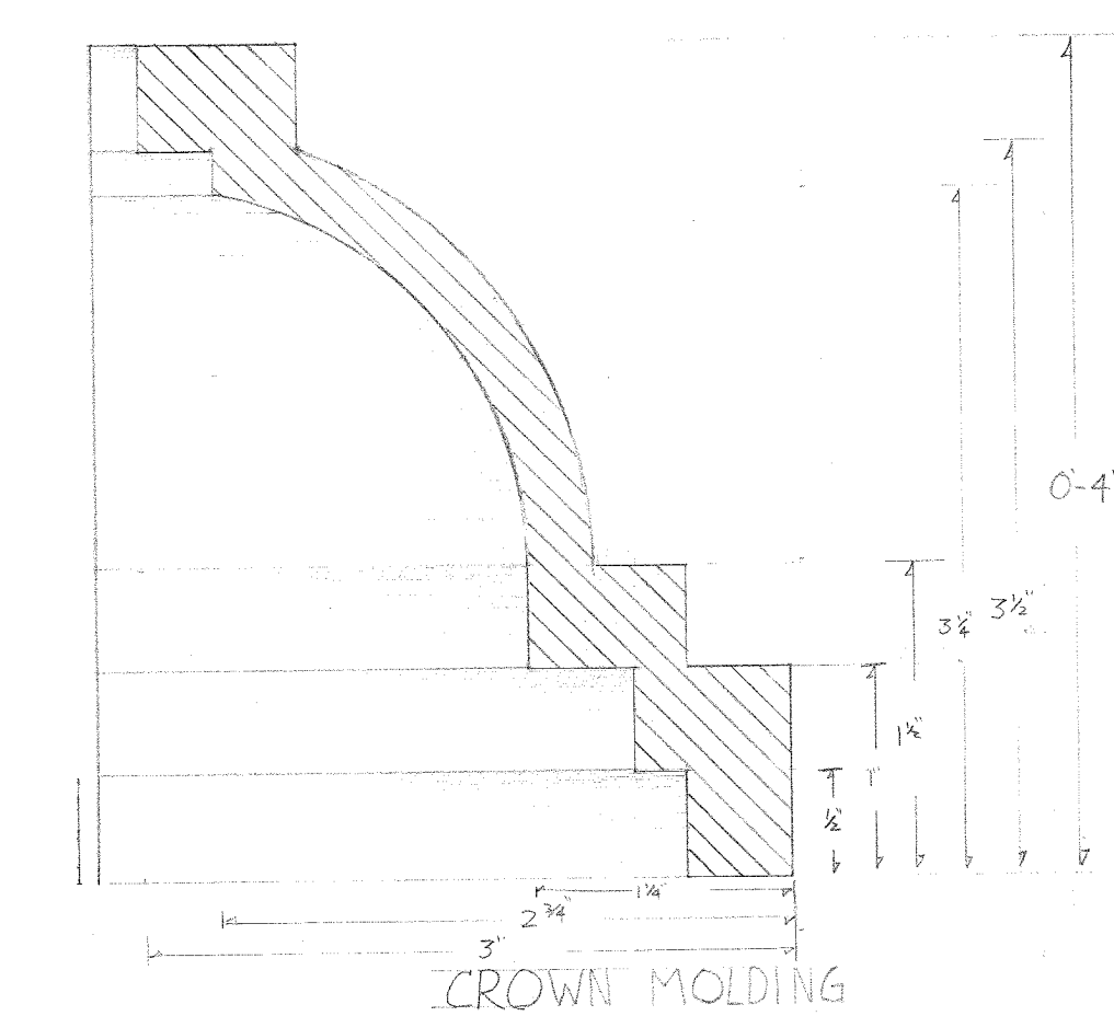
11 [DETAIL D] Scale: Actual Size
