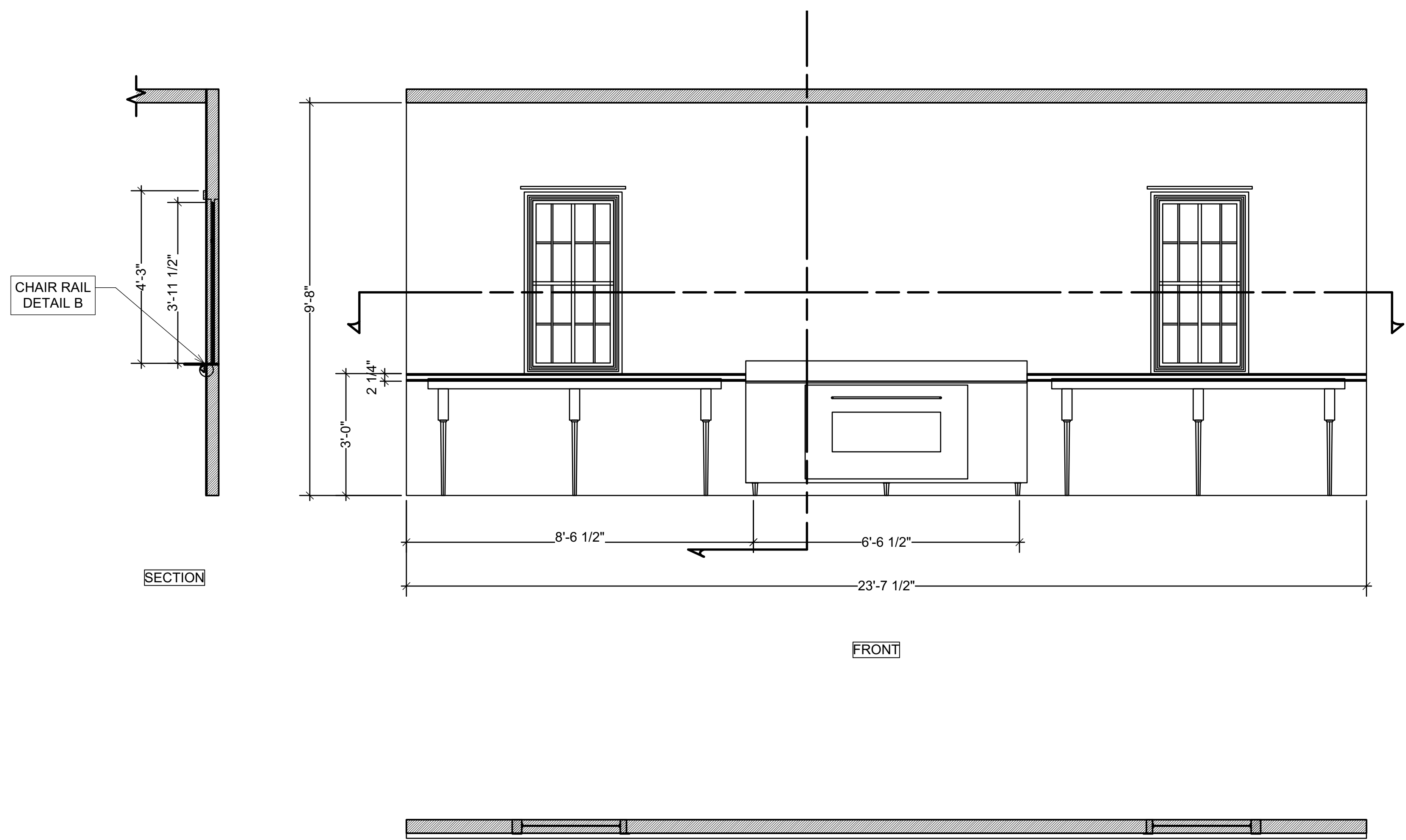
6 [KITCHEN WALL 6] Scale: 1/2" = 1'-0"
