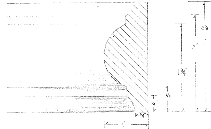
9 [DETAIL B] Scale: Actual Size
