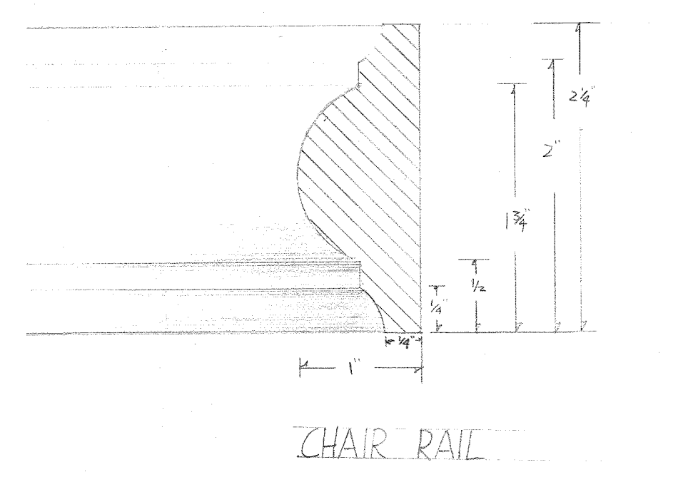
9 [DETAIL B] Scale: Actual Size
