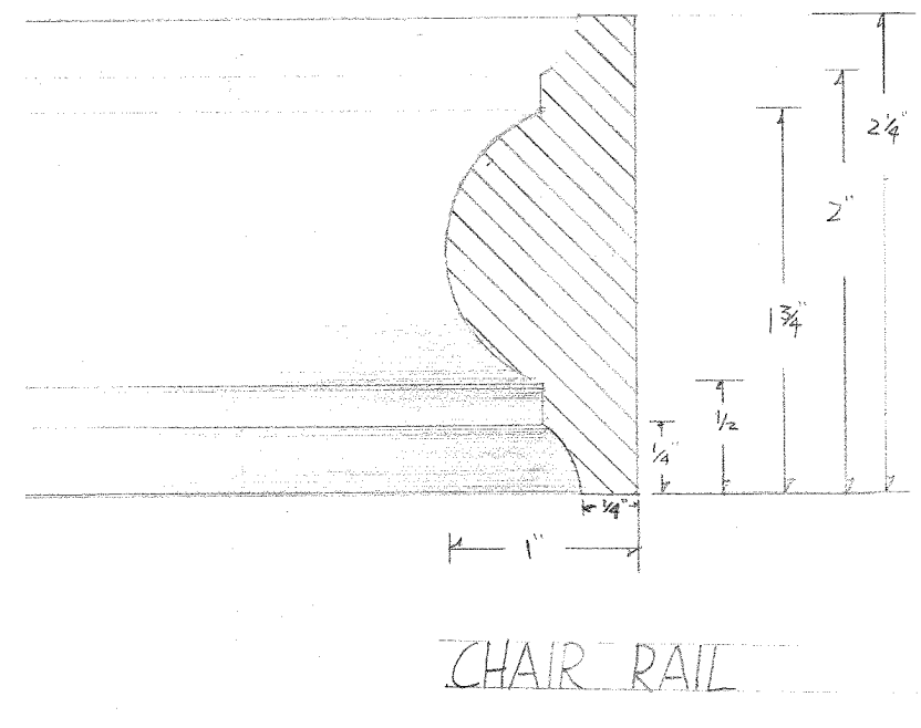
9 [DETAIL B] Scale: Actual Size
