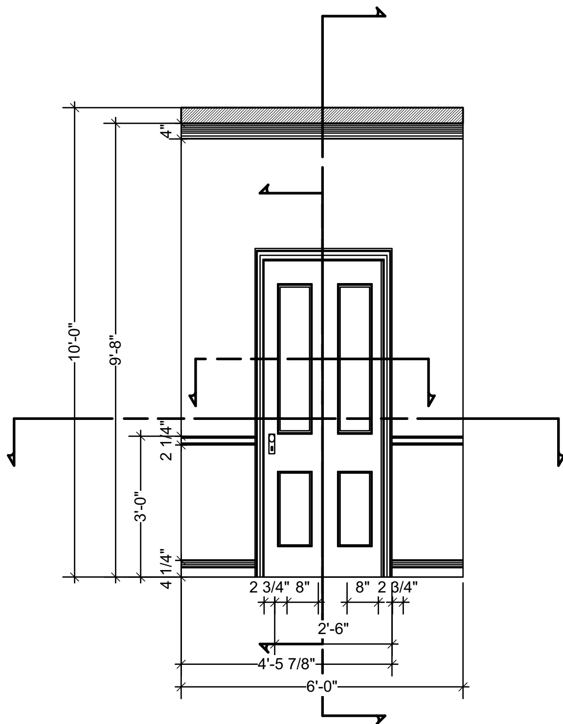
6 [FINZI ROOM WALL 6] Scale: 1/2" = 1'-0"
