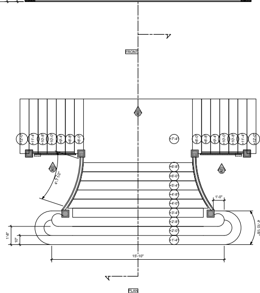
11 & A1 [ATRIUM GRAND STAIRCASE] Scale: 1/2" = 1'-0"
