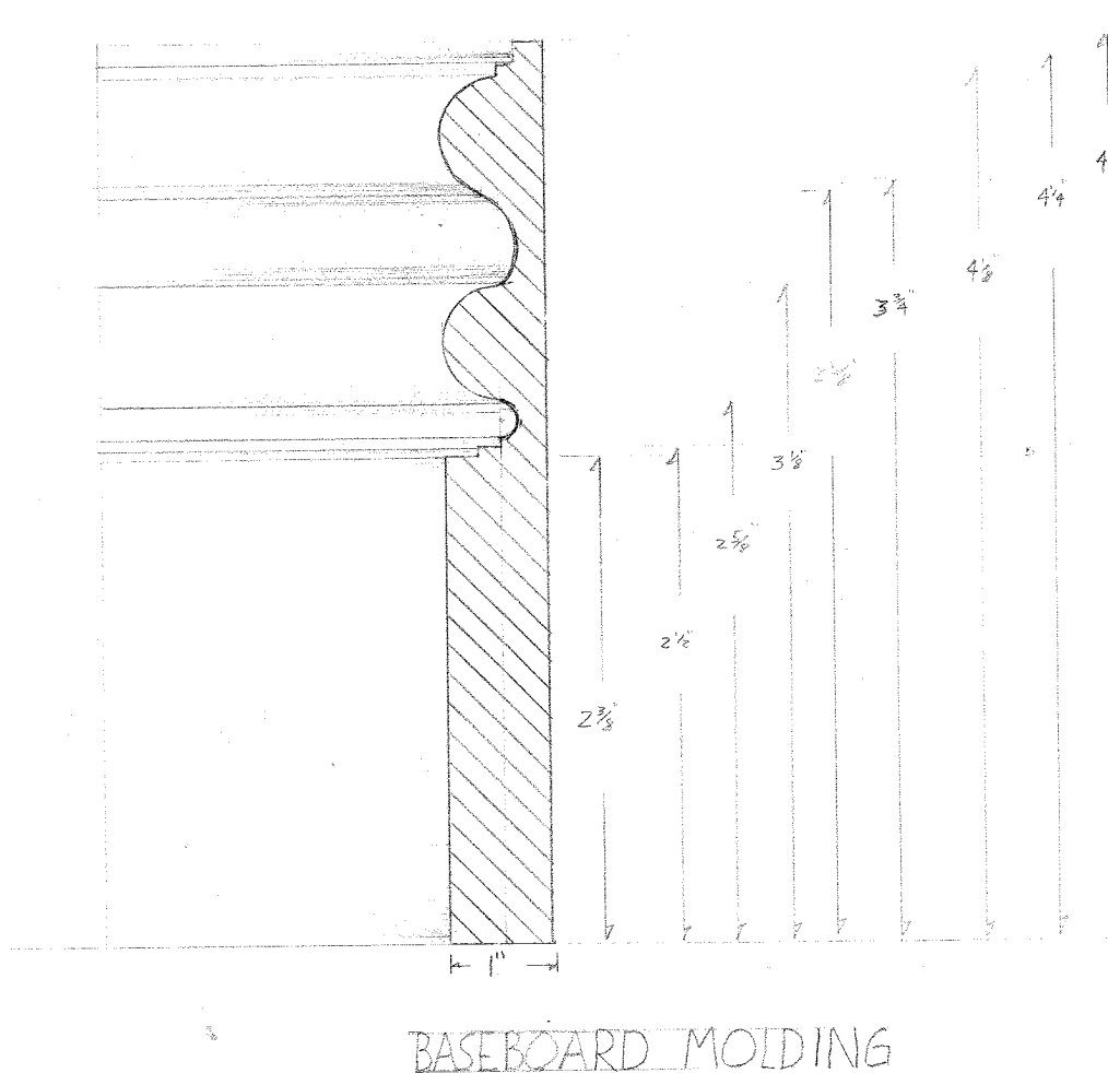
10 [DETAIL A] Scale: Actual Size
