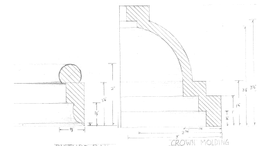
8 [DETAIL C] Scale: Actual Size
