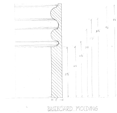
10 [DETAIL A] Scale: Actual Size
