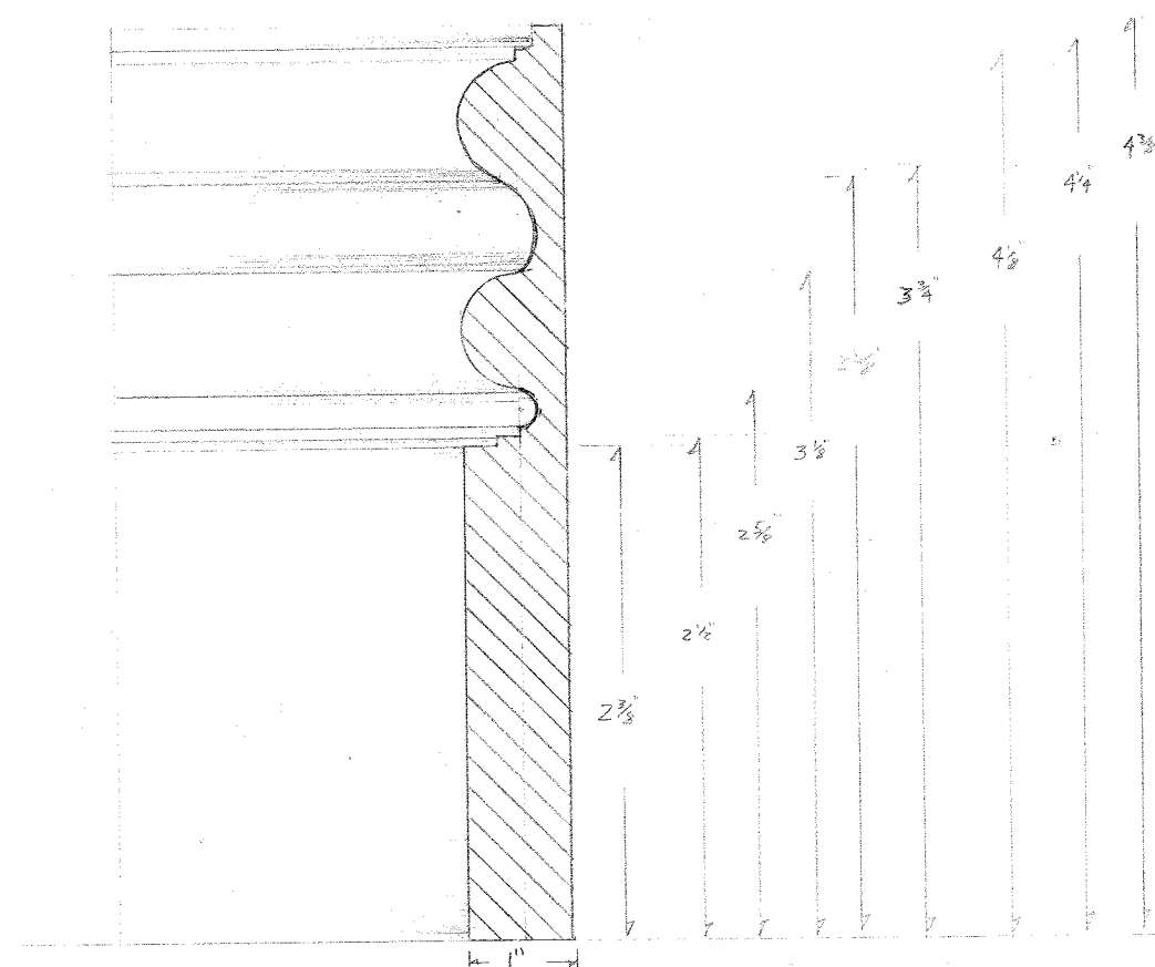
9 [DETAIL B] Scale: Actual Size
