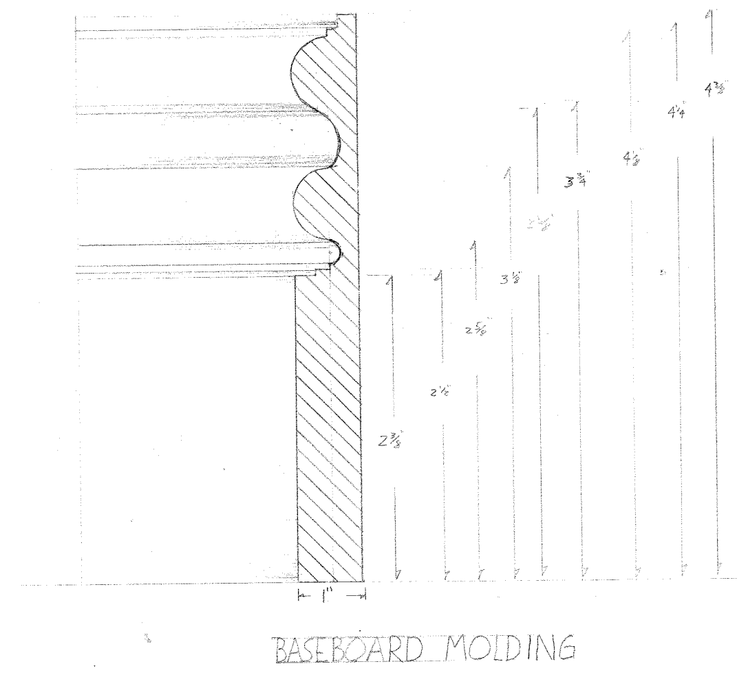
10 [DETAIL A] Scale: Actual Size
