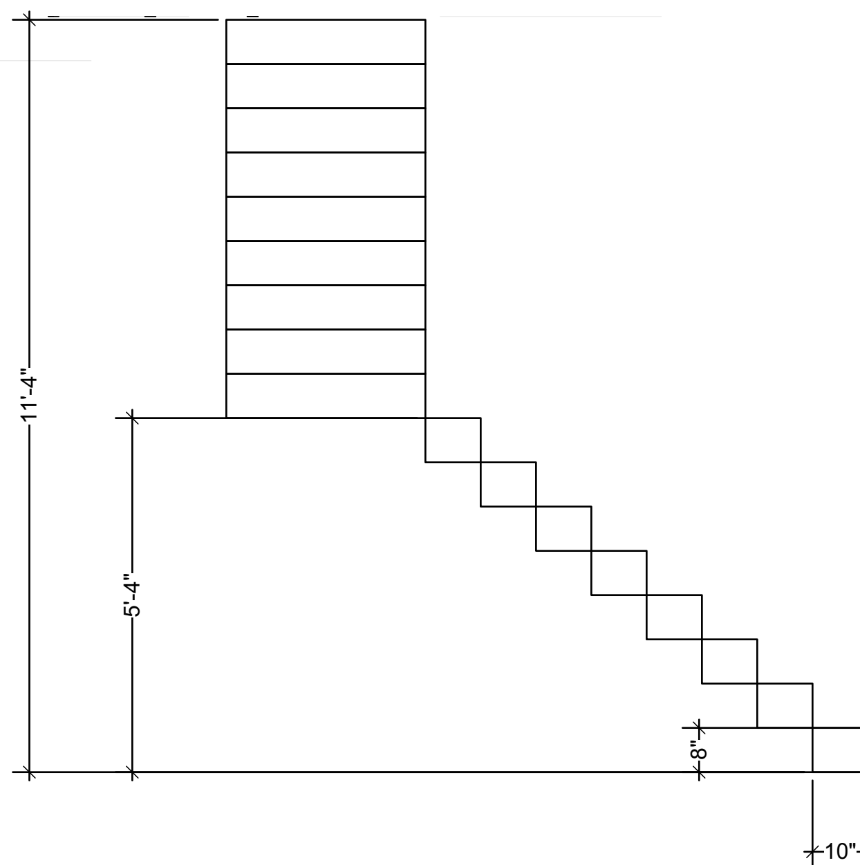
2 [FINZI STAIRS] Scale: 1/2" = 1'-0"
