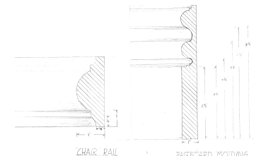
9 [DETAIL B] Scale: Actual Size
