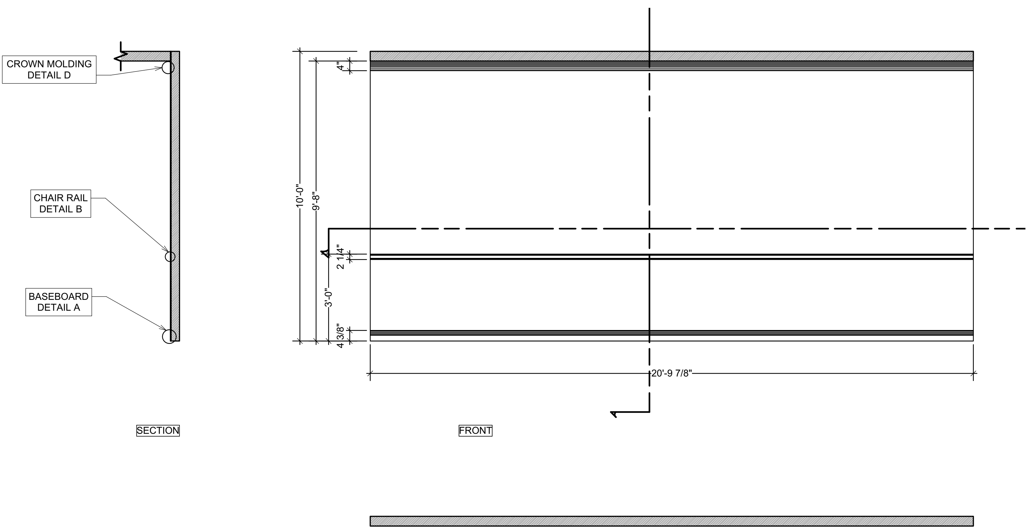
3 [DANTE ROOM WALL 3] Scale: 1/2" = 1'-0"
