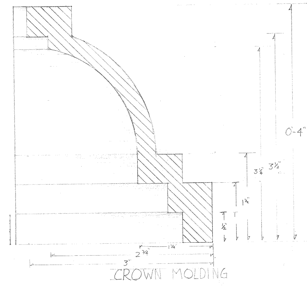
11 [DETAIL D] Scale: Actual Size
