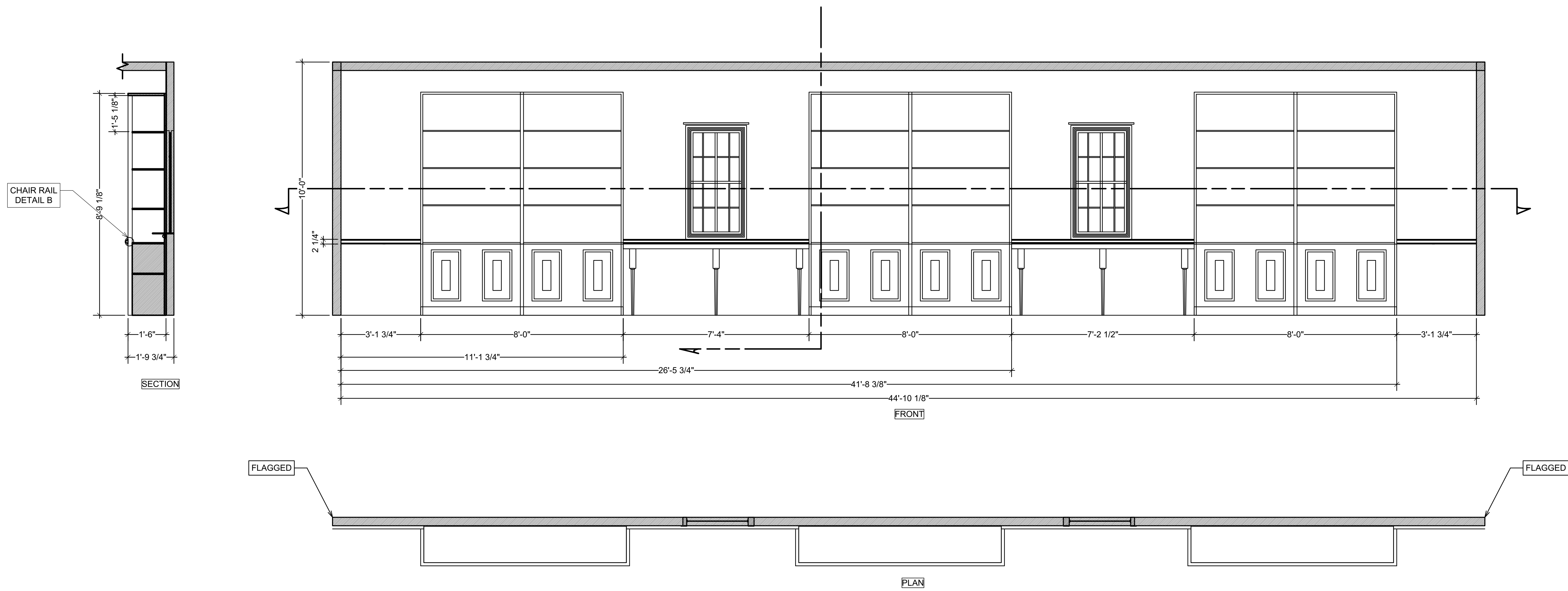
5 [KITCHEN WALL 5] Scale: 1/2" = 1'-0"
