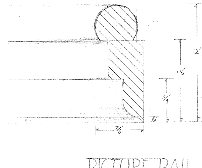
8 [DETAIL C] Scale: Actual Size
