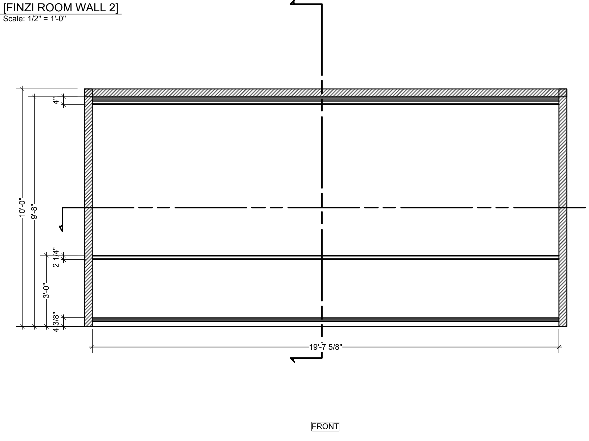
2 [FINZI ROOM WALL 2] Scale: 1/2" = 1'-0"
