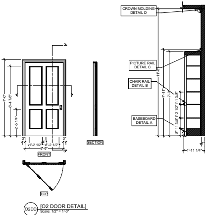
O2DO [O2 DOOR DETAIL] Scale: 1/2" = 1'-0"
