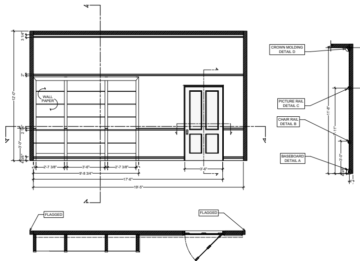
O1 [ORATORIO WALL ELEVATION] Scale: 1/2" = 1'-0"
