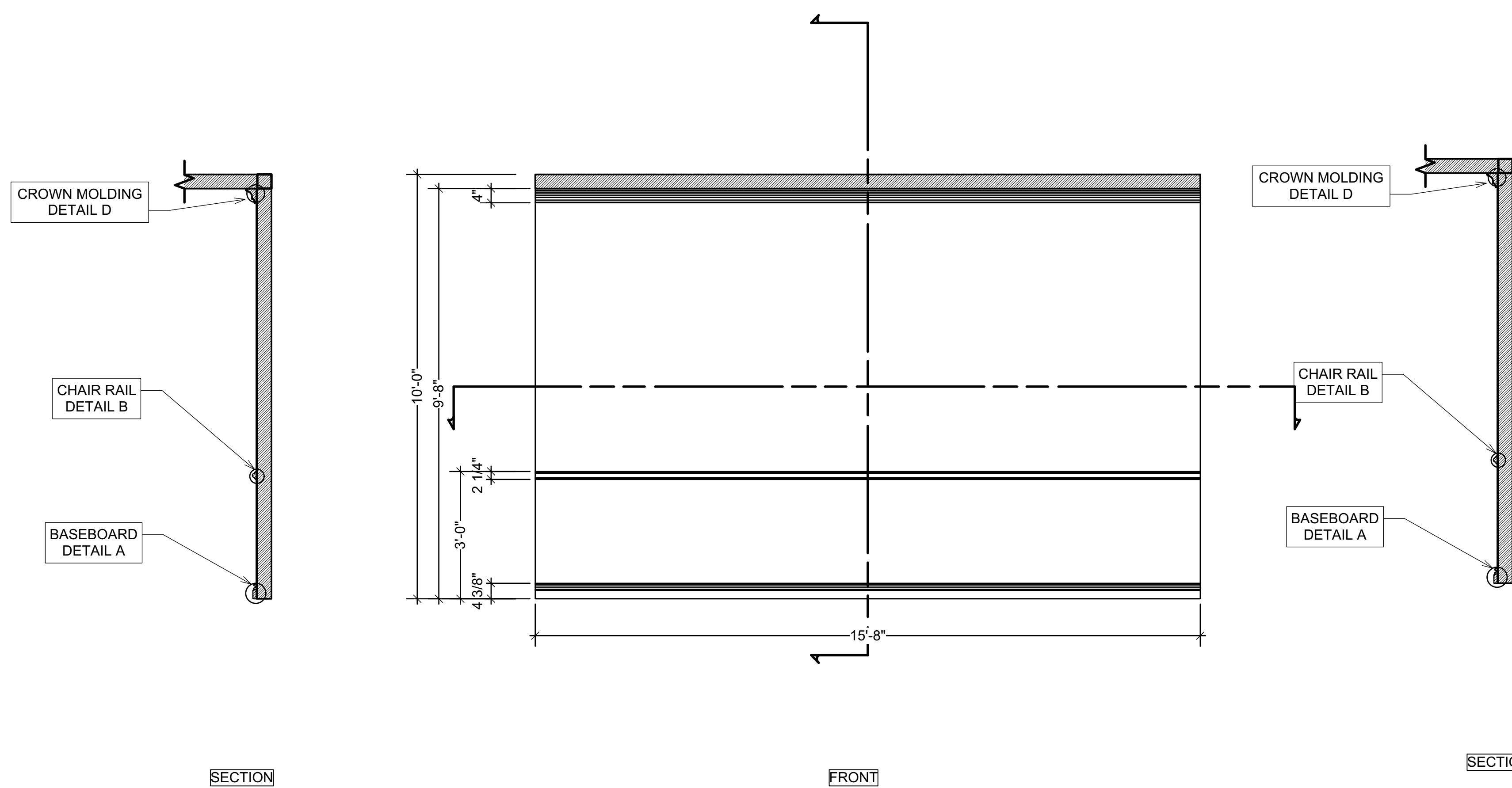
1 [FINZI RM WALL 1] Scale: 1/2" = 1'-0"
