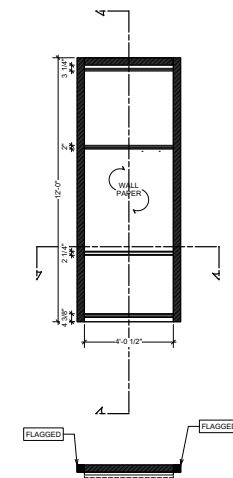
O8 [DETAIL C] Scale: Actual Size
